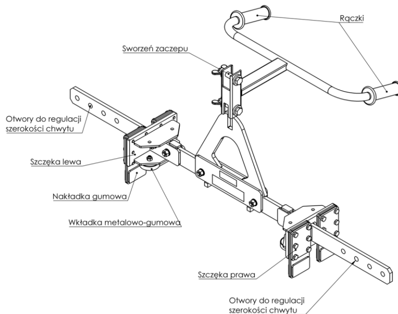
Rys.1 Objaśnienie elementów ustawczych narzędzia
