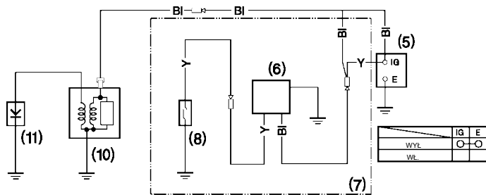
Wersja z systemem Oil Alert®, bez rozrusznika elektrycznego
