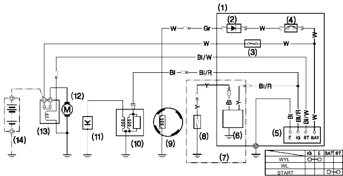
Wersja z systemem Oil Alert® i rozrusznikiem elektrycznym
