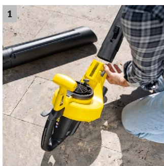
1 Rury ssące i nadmuchowe można odpinać osobno
